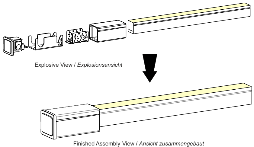
Finished Assembly View / Ansicht zusammengebaut
